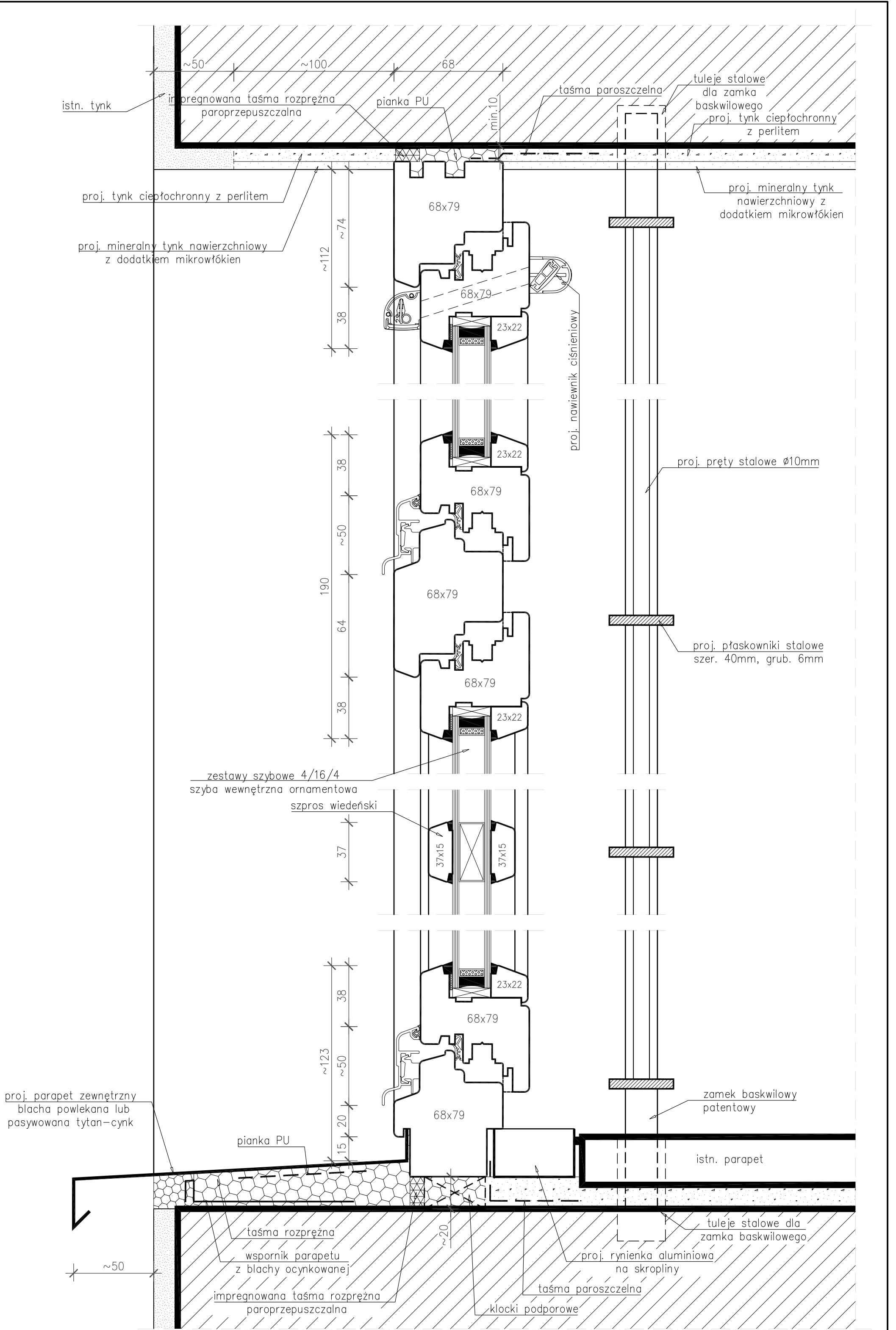
SCHEMAT ROZWIĄZAŃ OKIEN ZAKRYSTII przekrój pionowy
