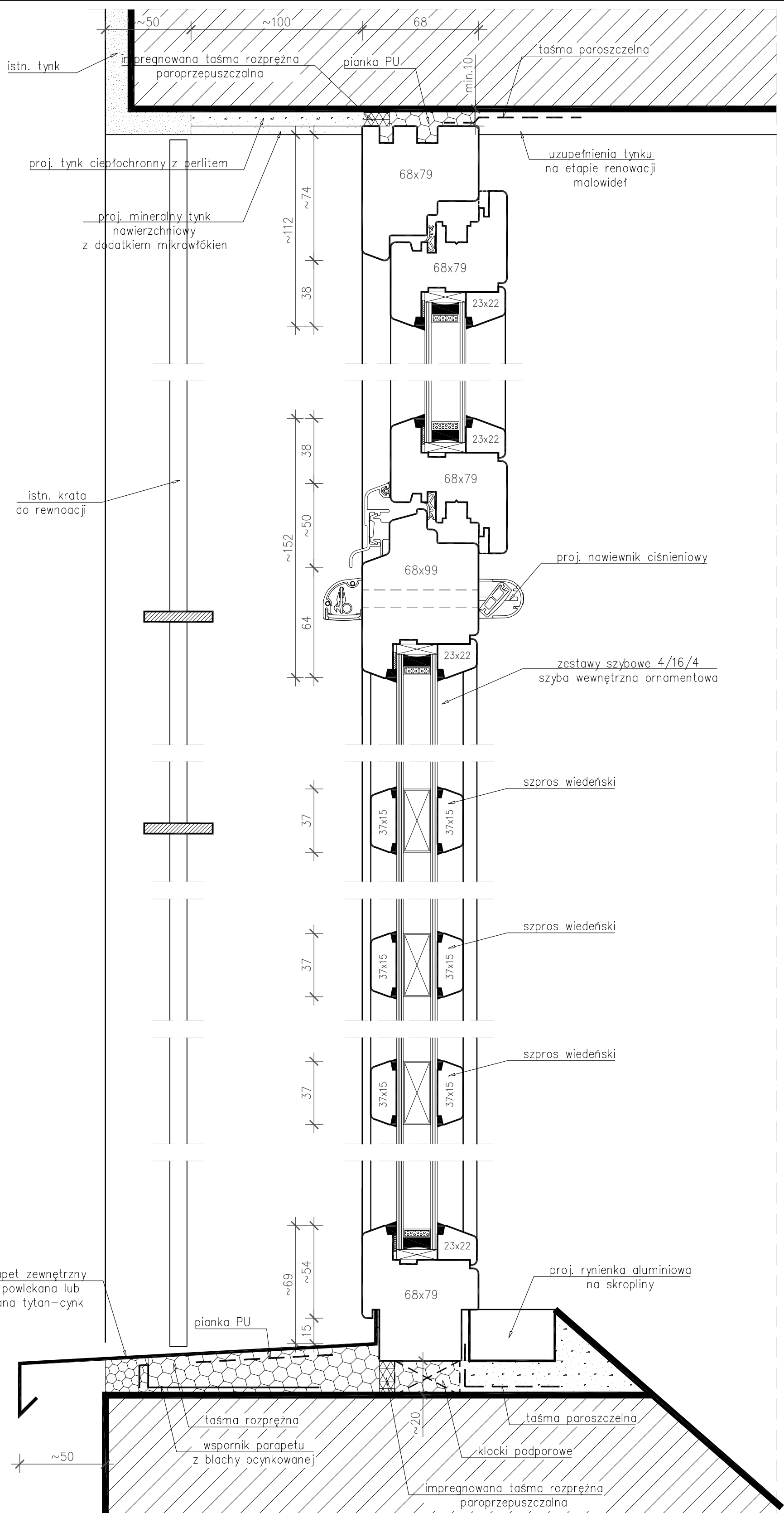
SCHEMAT ROZWIĄZAŃ OKIEN KOŚCIOŁA przekrój pionowy
